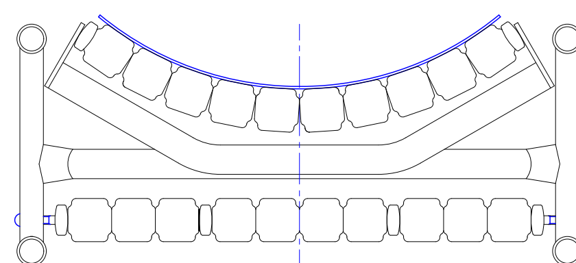
中間部断面図
